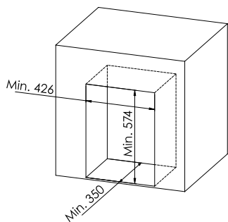
Modello a pavimento e modello a parete Inspire
