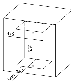
Modello nascosto a parete Inspire
