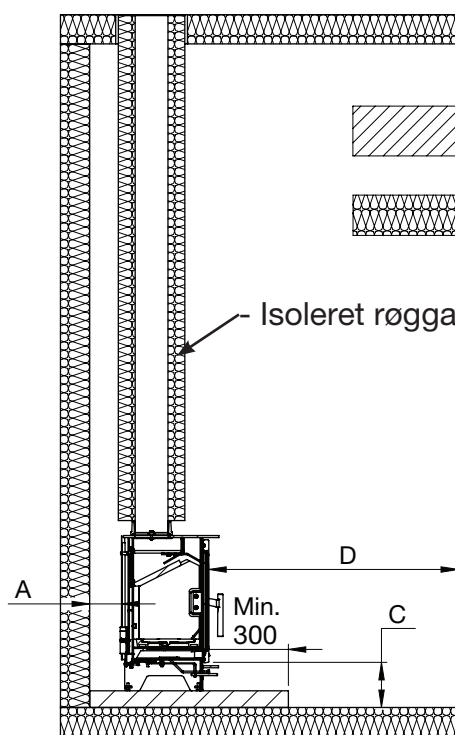
Snit A-A
