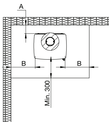
Snit B-B
