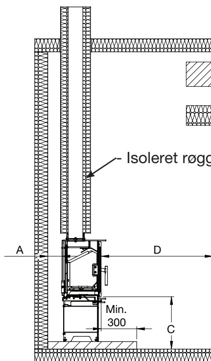
Snit A-A
